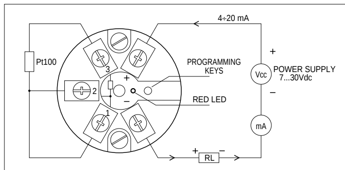
Fig. 2 Schéma de branchement et programmation des transmetteurs.
