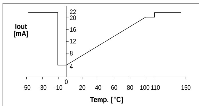
Fig. 1 Gamme 0...100°C, courant de sortie par rapport à la température.
