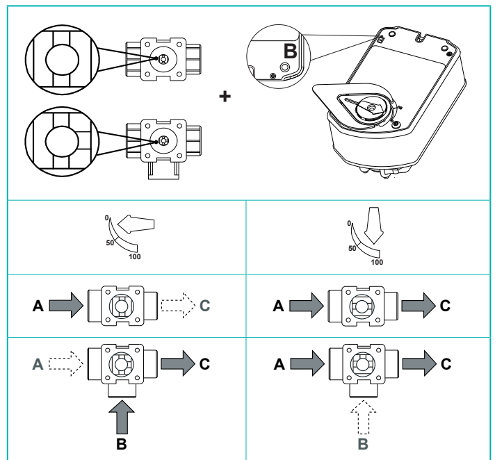
Figure 7 : Normalement Fermé (le ressort ferme la vanne)
