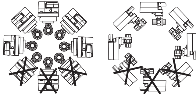
Figure 5 : Positions de Montage pour l'Eau Refroidie et pour Applications avec Atmosphère Condensante
