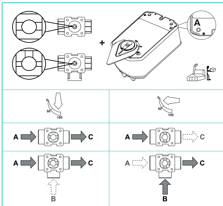
Figure 6 : Normalement Ouvert (le ressort ouvre la vanne)
