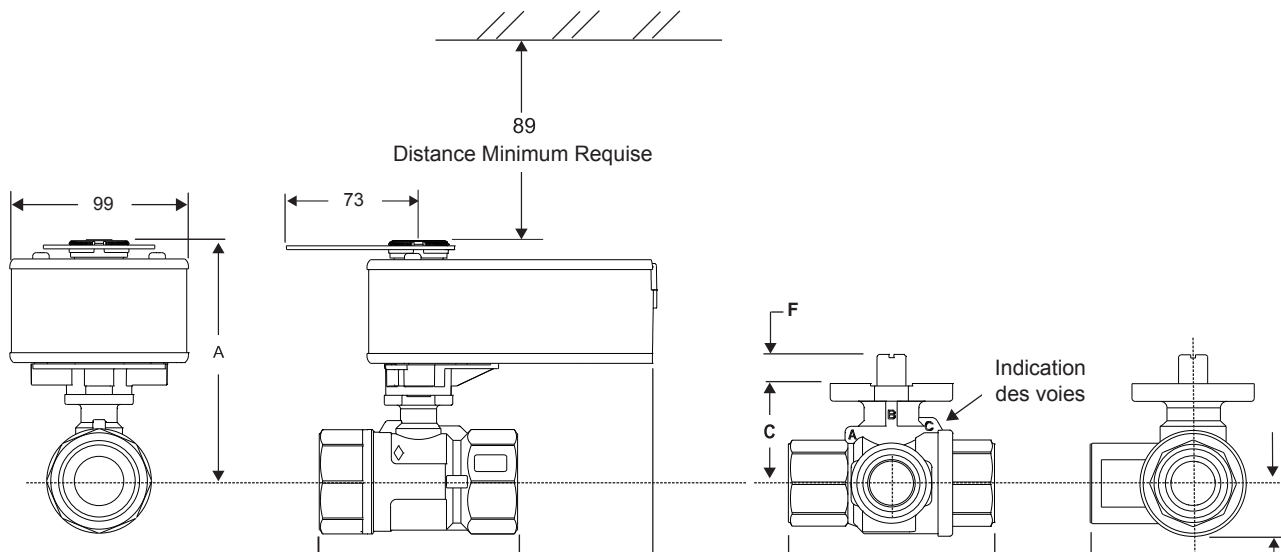
Figure 8 : Servomoteurs avec ressort de rappel BxFx.08(S) et vannes à boisseau sphérique JV205 et JV305
