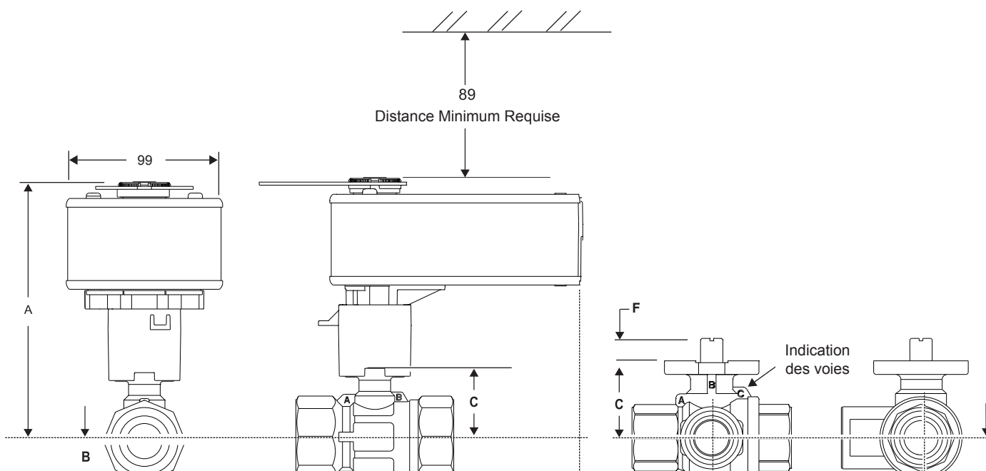
Figure 9 : Servomoteurs avec ressort de rappel BxFx.08(S), vannes à boisseau JV205 et JV305 et barrière thermique
